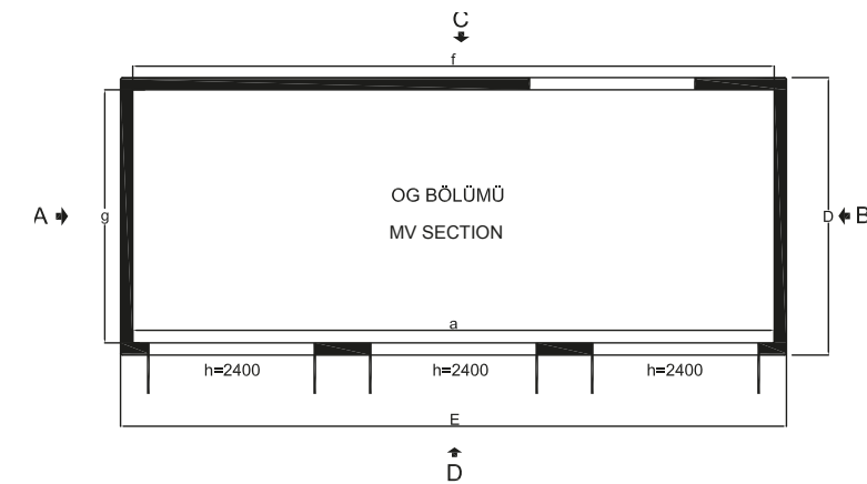
ABK-H HAVA YALITIMLI HÜCRELİ DAĞITIM MERKEZLERİ
