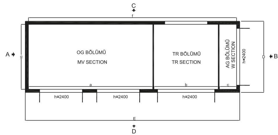
ABK-B HAVA YALITIMLI HÜCRELİ KOMPAKT TRAFİ MERKEZLERİ (1600 kVA)
