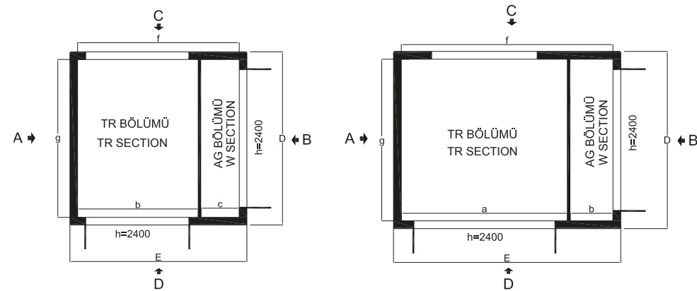
ABK-T AG PANO VE DAĞITIM TRANSFORMATÖRLÜ MERKEZLER
