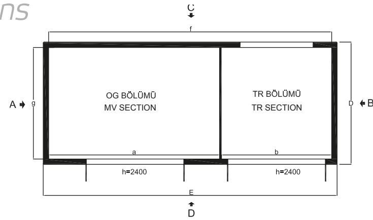
ABK-D AG PANOSUZ HAVA YALITIMLI HÜCRELİ KOMPAKT TRAFİ MERKEZLERİ (1600 kVA)
