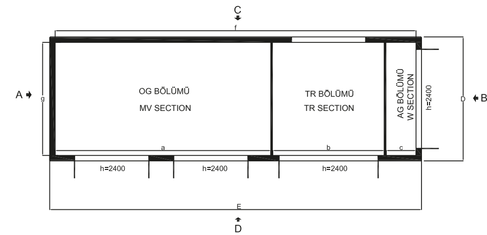
ABC-C AG PANOSUZ HAVA YALITIMLI HÜCRELİ KOMPAKT TRAFİ MERKEZLERİ (1000 kVA)
