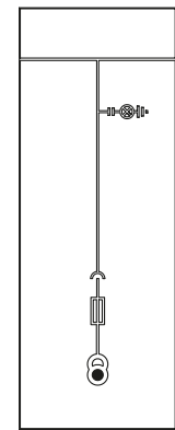
Gerilim Ölçü Hücresi Voltage Measurment Switchgear
