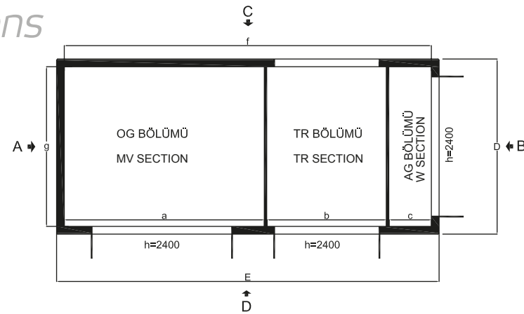
ABK-A HAVA YALITIMLI HÜCRELİ KOMPAKT TRAFİ MERKEZLERİ (1000 kVA)
